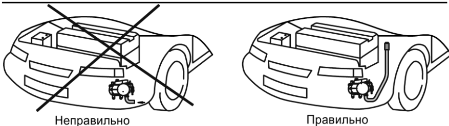
Рис.7.4 – Монтаж подогревателя за бампером.
