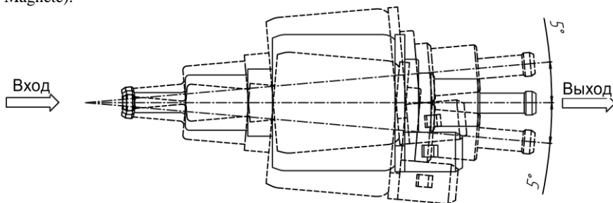
Рис. 7.8 Допустимое монтажное положение топливного насоса (производства Thomas Magnete)
