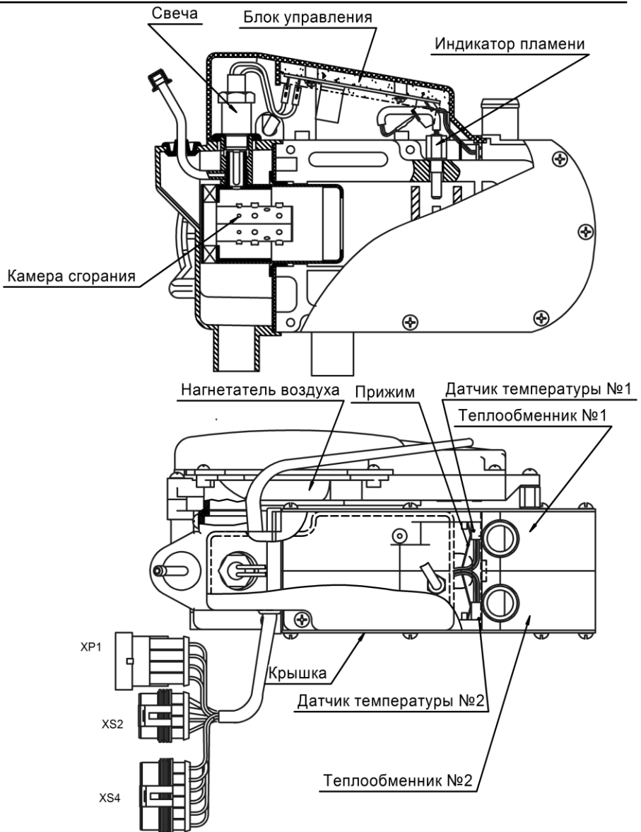
Рис 4.3- Основные узлы нагревателя
