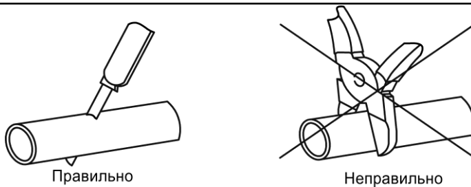
Рис. 7.9 - Отрезка трубопровода перед установкой.
