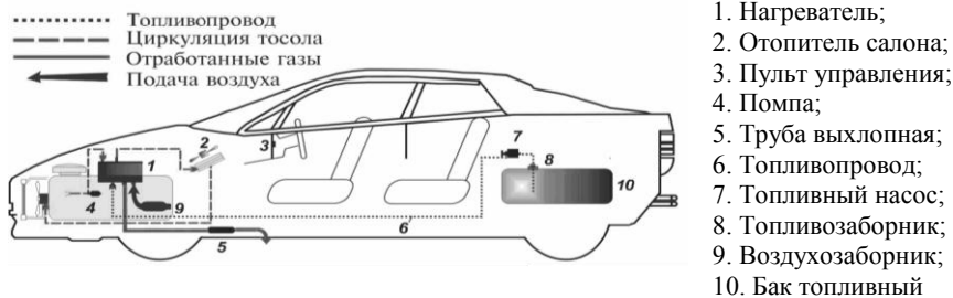
Рис. 7.1- Схема установки подогревателя на автомобиль
