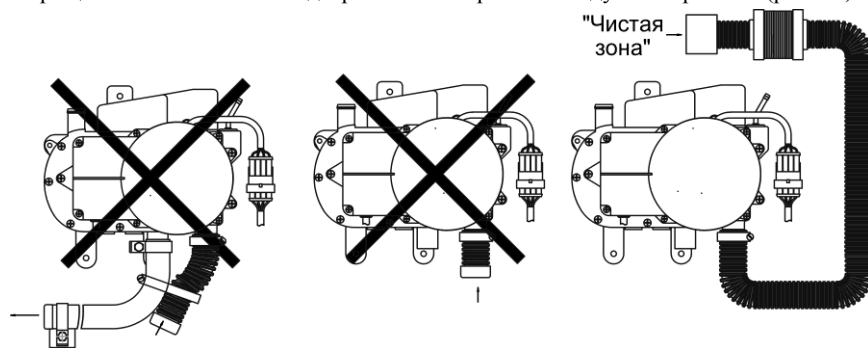
Рис.7.3 – Монтаж воздухозаборника.
