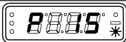
Рис. 6.13 – Индикатор при работе подогревателя в режиме розжига.
