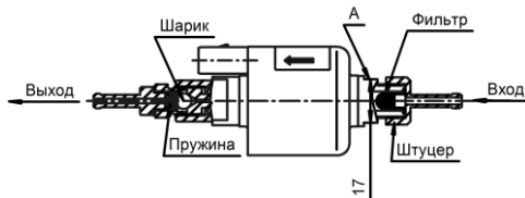
Рис. 9.1 – Топливный насос
