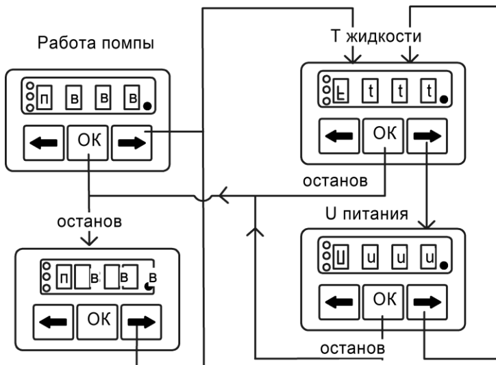
Рис. 6.29 – Схема работы с пультом при работе помпы.
