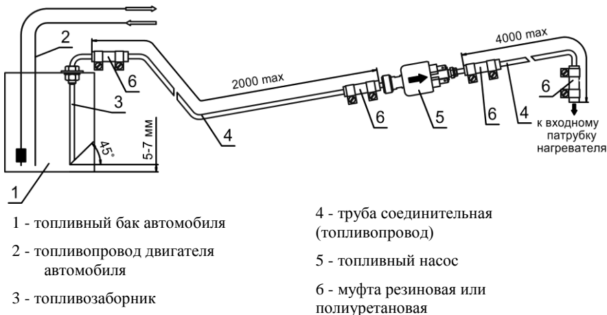
Рис. 7.6 - Схема присоединения топливопровода к узлам подогревателя
