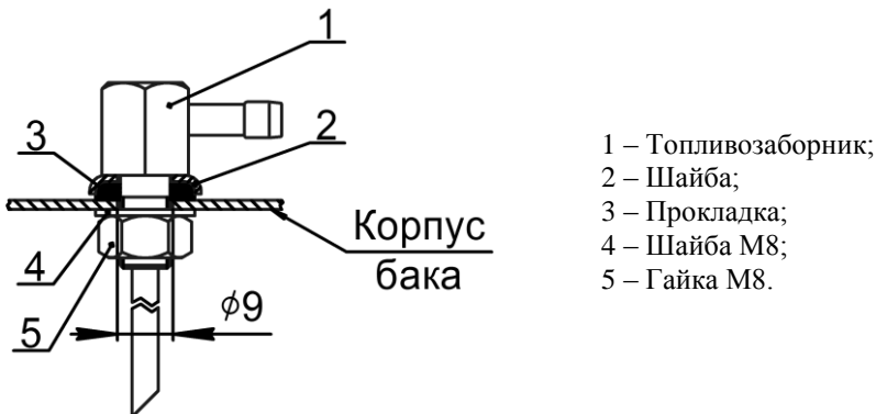
Рис. 7.5 – Монтаж топливозаборника
