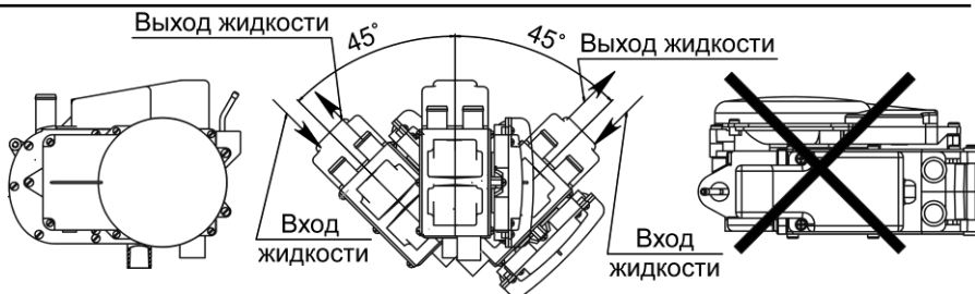
Рис. 7.2- Допустимые рабочие положения нагревателя
